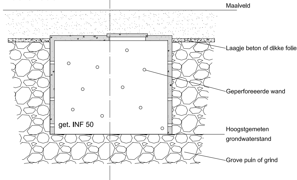
Doorsnede
