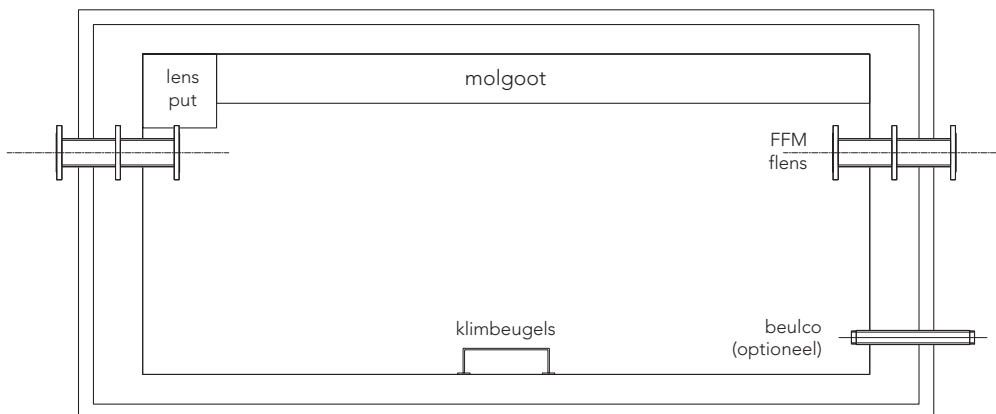
Bovenaanzicht put
