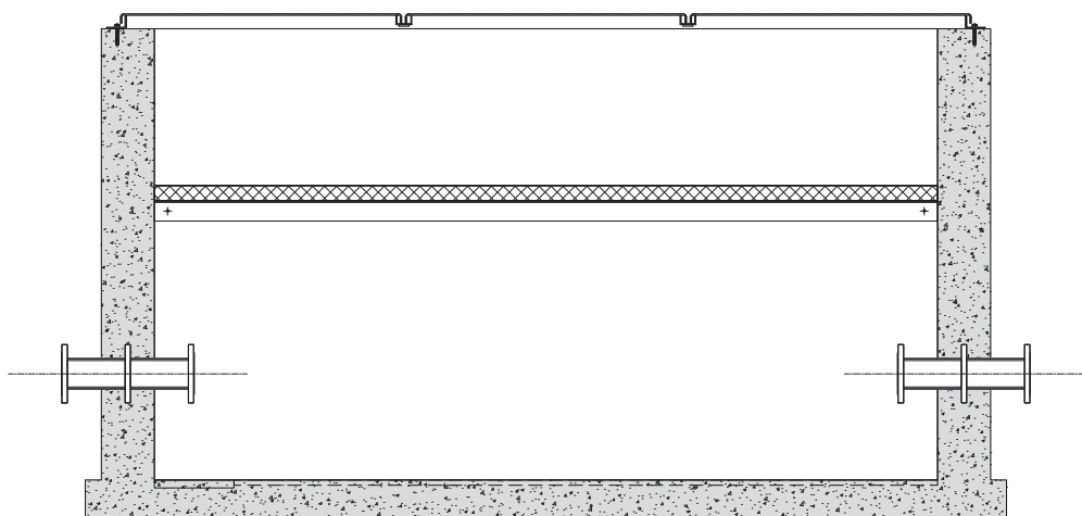
Doorsnede
