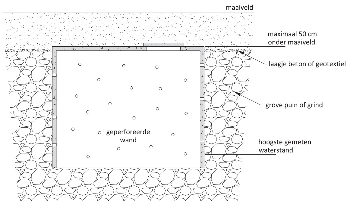
doorsnede
