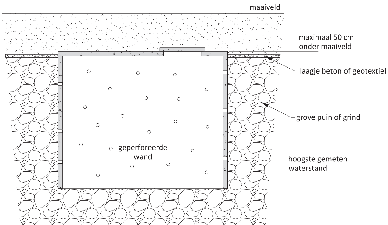
doorsnede
